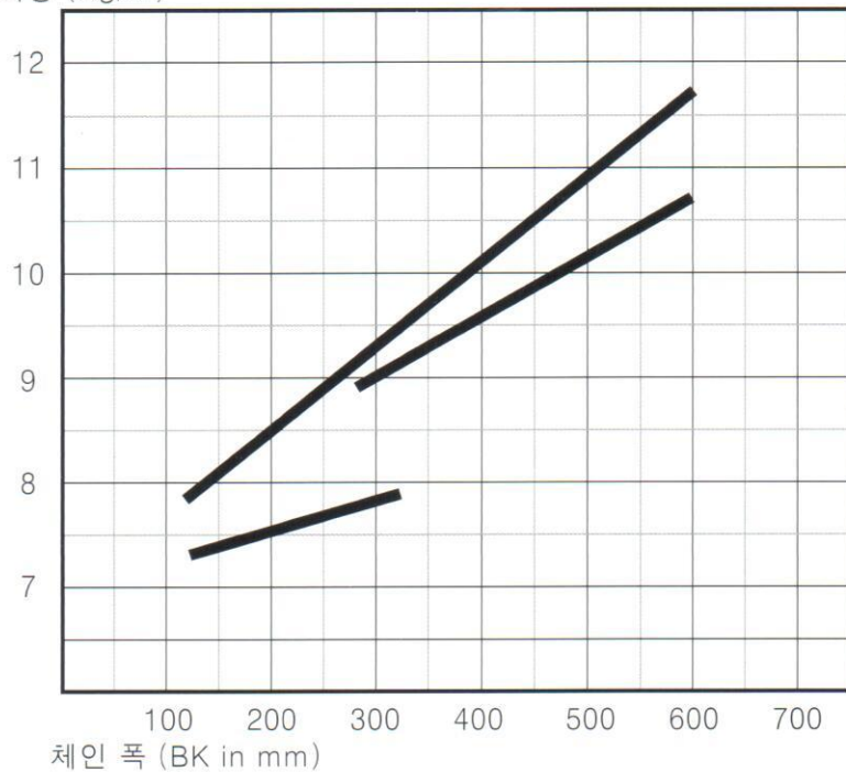
체인사하중 (Kg/m)
