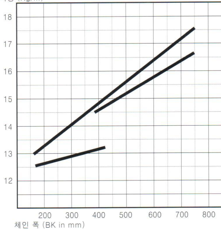
체인사하중 (Kg/m)
