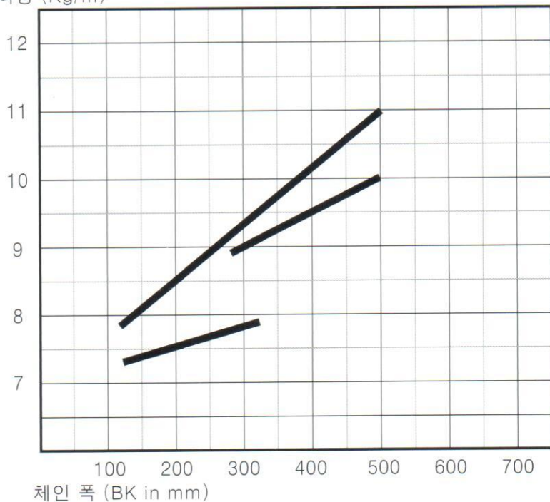
체인사하중 (Kg/m)
