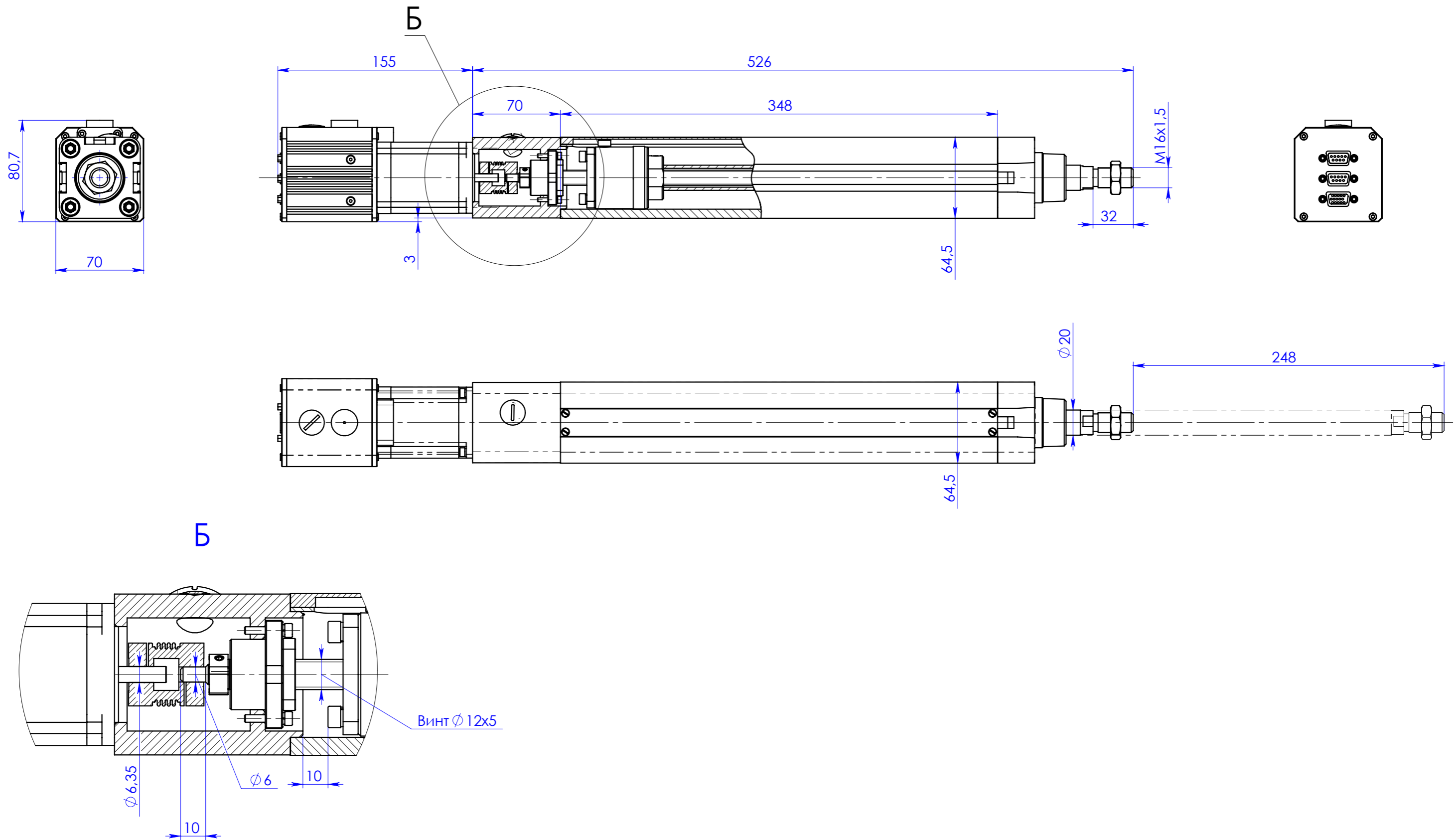
Общий вид модулей линейного перемещения ШМ-2
