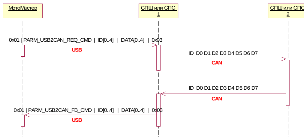
Рис. 5. Режим ретрансляции USB в CAN.
