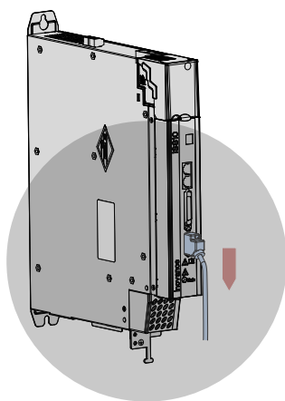
图 2-10 线缆走线要求示意图
