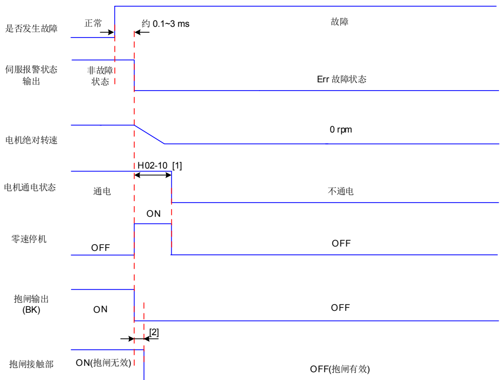
d) 第 2 类故障 带抱闸：强制为零速停机，保持自由运行状态
