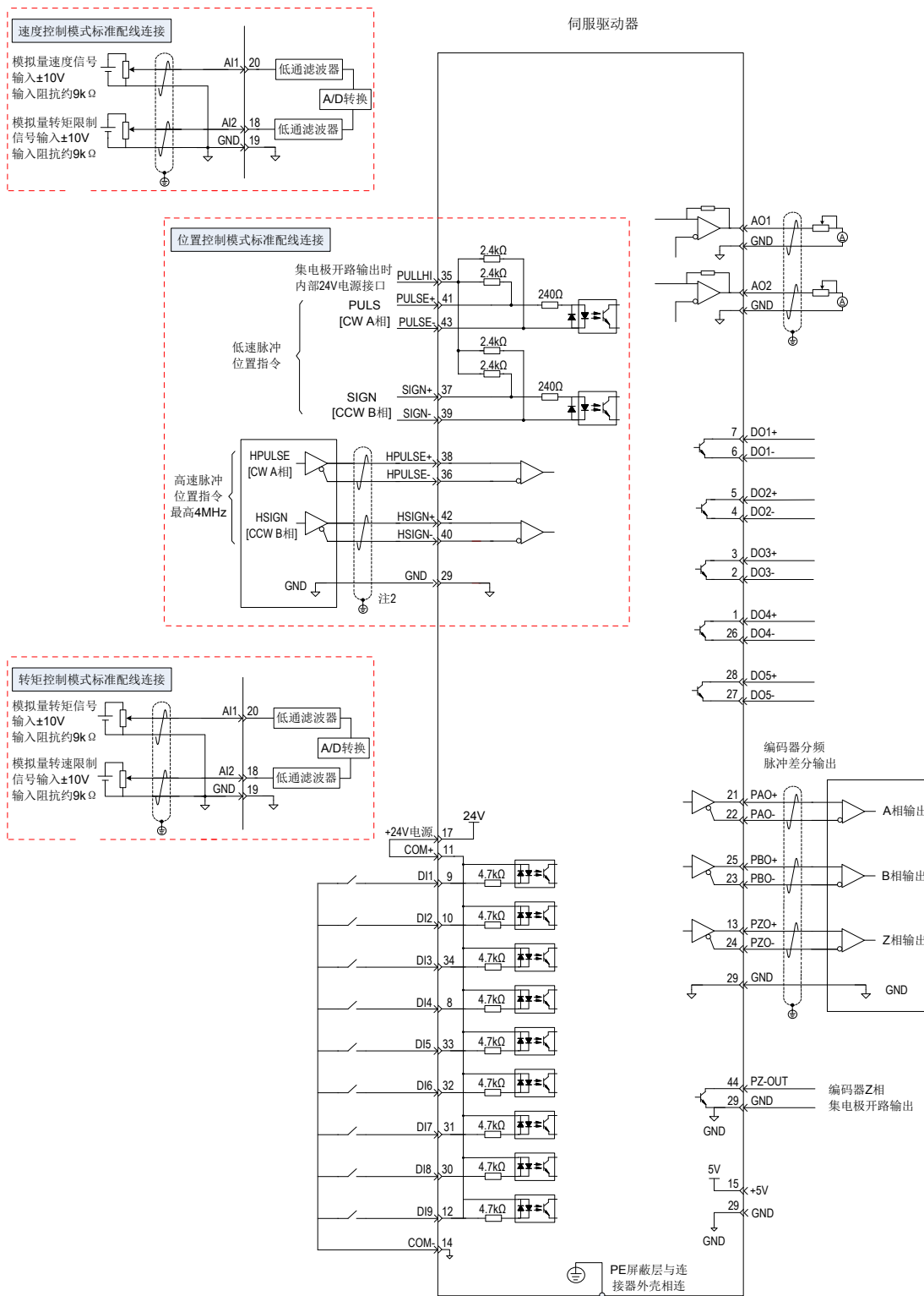
图 3-15 三种控制模式配线图举例
