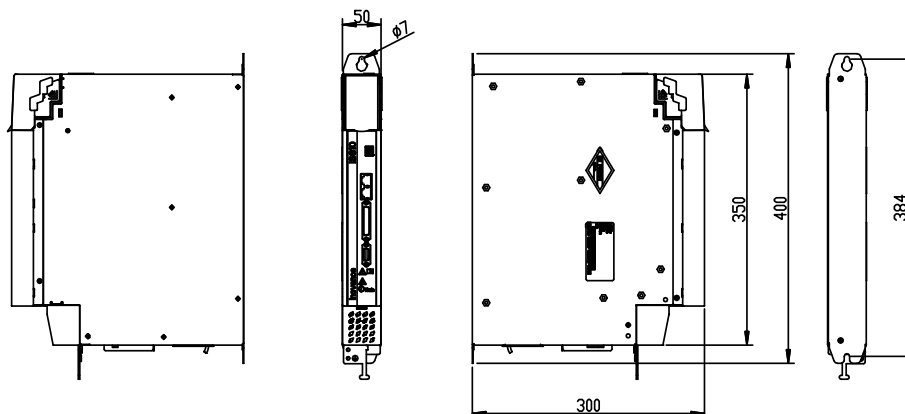
图 2-3 IS810P50M4T***** (SIZE 1) 外形尺寸图
