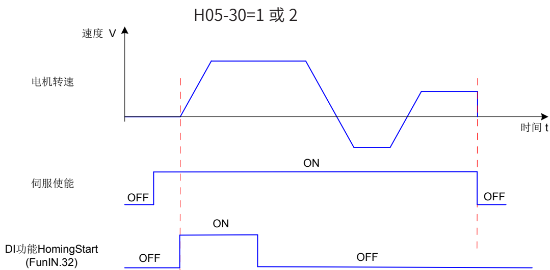
图 5-56 时序图举例
