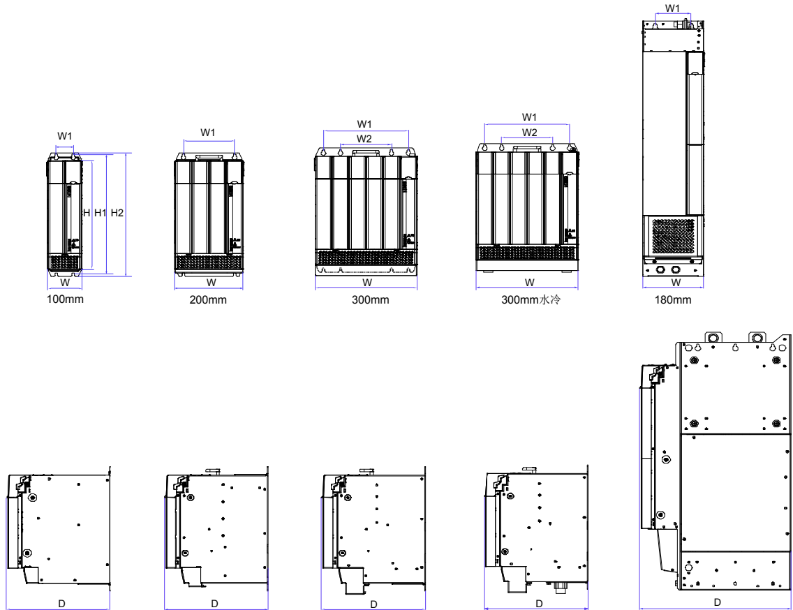
图 2-2 MD810-20M4T**G*** 外型尺寸示意图
