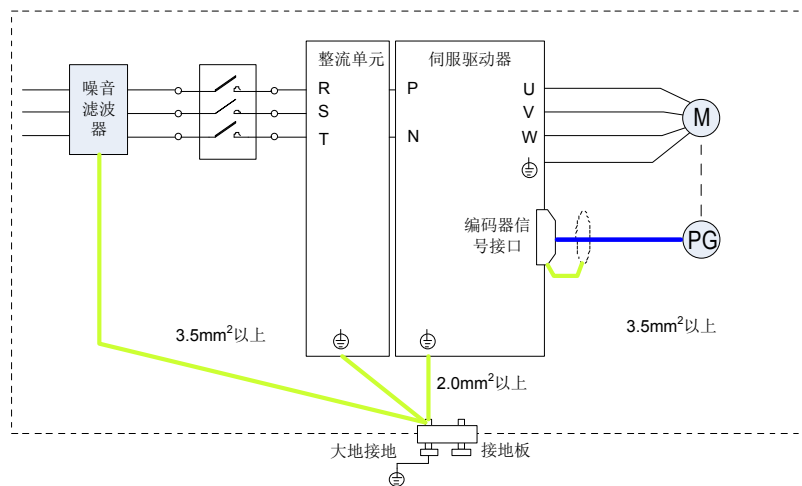
图 3-33 抗干扰配线实例
