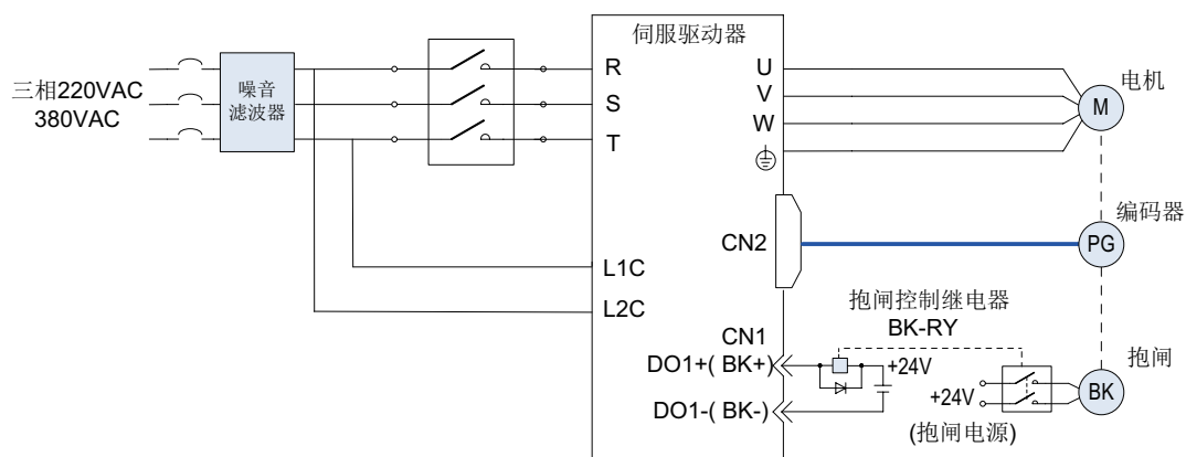
图 3-18 抱闸配线图
