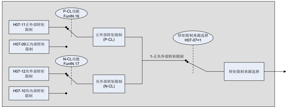
图 5-90 H07-07=1 转矩限制来源
