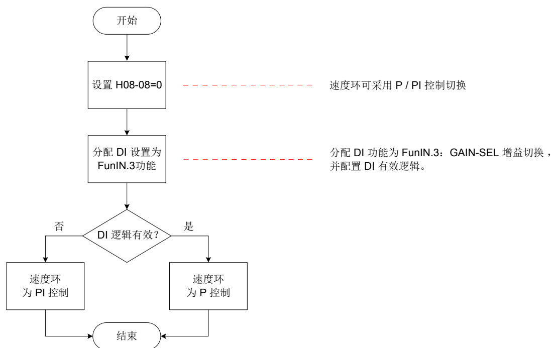
图 6-7 H08-08=0 增益切换流程图
