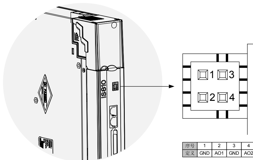
图 3-32 模拟量监视信号连接器端子
