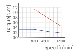
X6MH010H ▲
