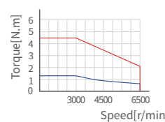
X6MH040A ▲
